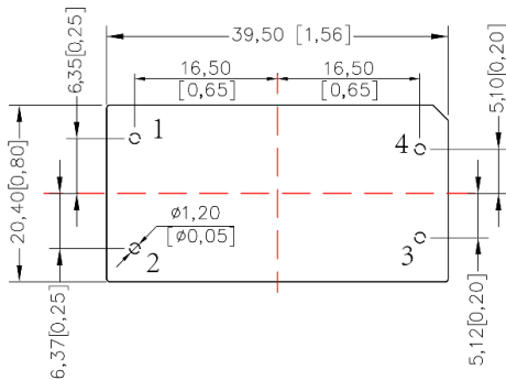
PCB封装参考尺寸图 (顶视)
