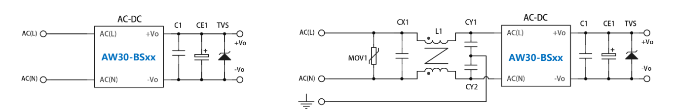
图 1 一般要求应用电路
