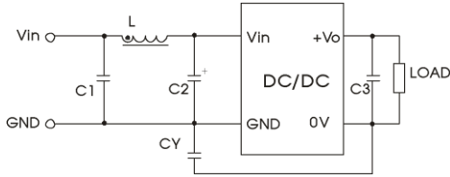
(图 2) EMC 推荐电路
